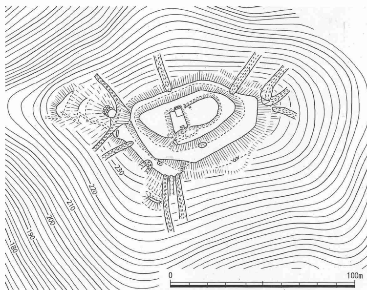
▲青佐山城跡縄張り図（上が北） 『岡山県中世城館跡総合調査報告書』第2冊－備中編－ 2020より
