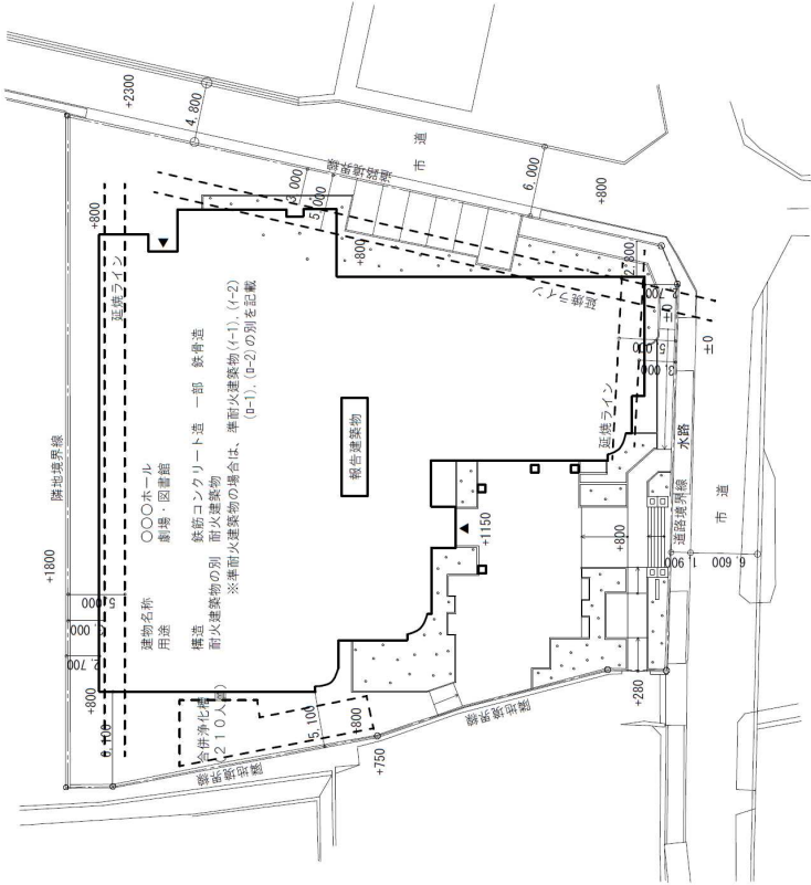
配置図 S = 1 / 800
