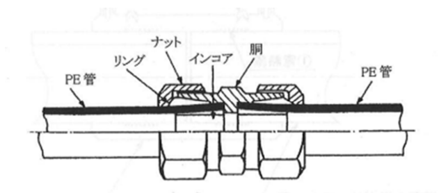
図2-22 水道用ポリエチレン管金属継手（JWWA B 116）の接合方法
