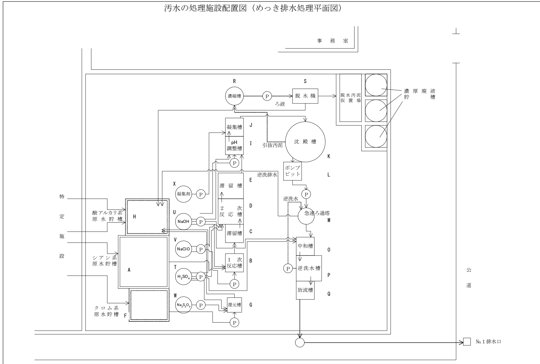
添付図-3 (2) 汚水の処理施設配置図の例 (2/2)
