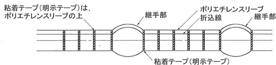
継手部
