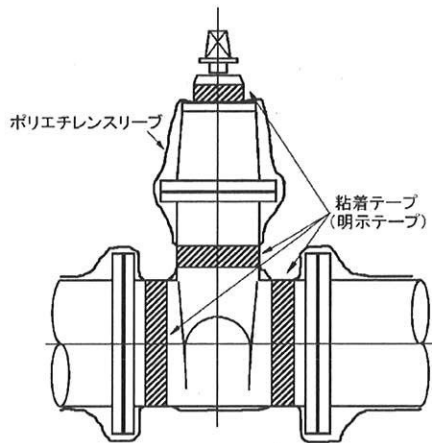
仕切弁部
