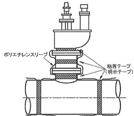
消火栓部
