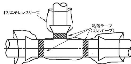
分岐部
