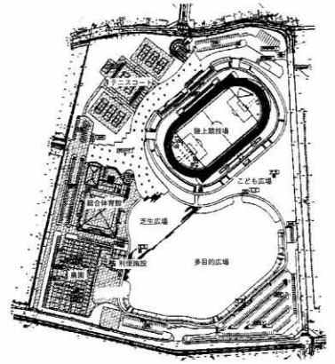
笠岡総合スポーツ公園計画平面図
